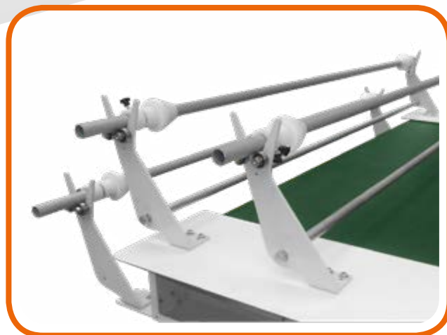
Attrezzatura carico rotoli tessuto Equipment for rolls loading
